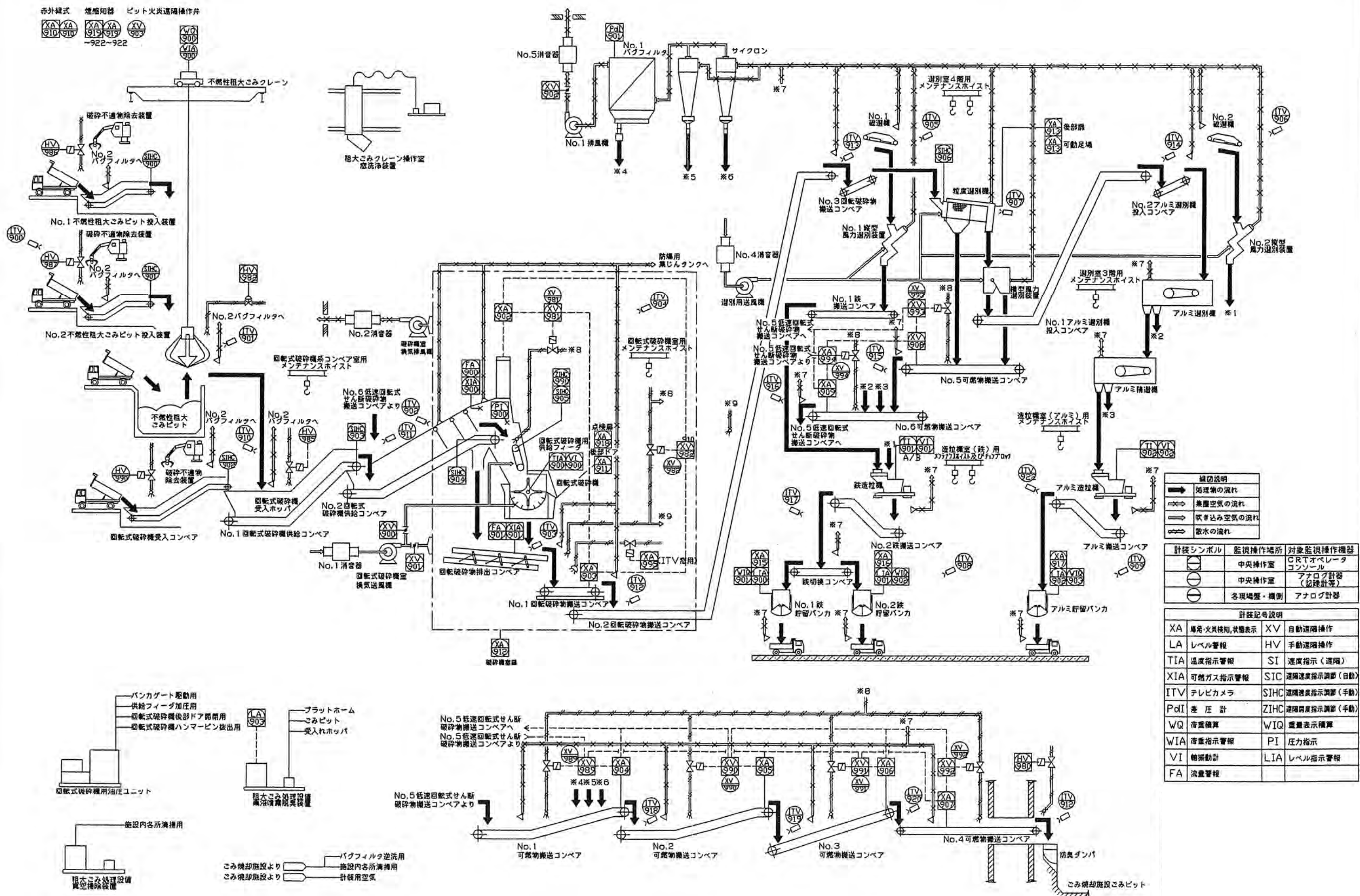
不燃性粗大ごみ処理フローシート
