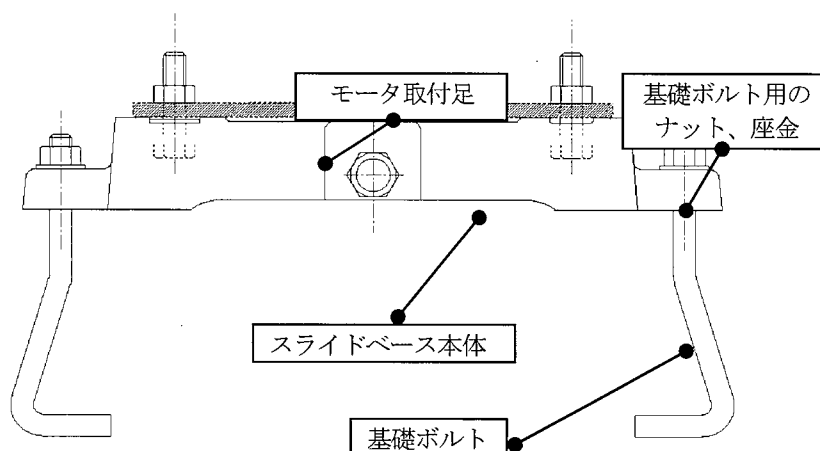
図1. スライドベースへの基礎ボルト取付例
