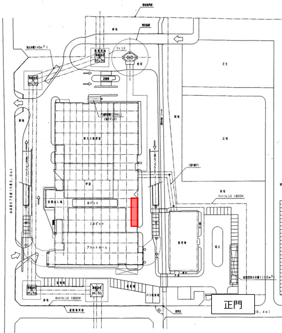
建物配置図
